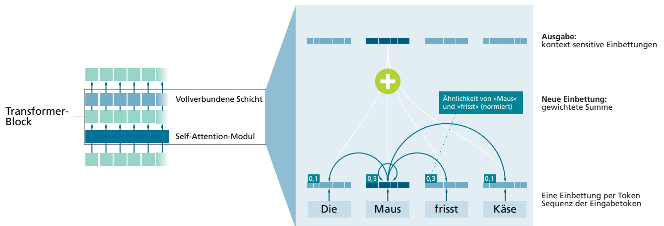
Abbildung 2: Der Transformer-Block besteht aus einem »Self-Attention-Modul«, das jedes Token mit allen anderen Token vergleicht. Quelle: Fraunhofer IAIS
